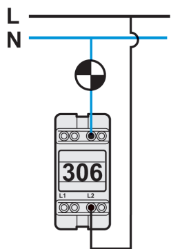
Interrupteur
