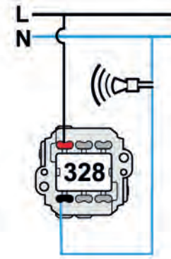
Bouton-poussoir rotatif
