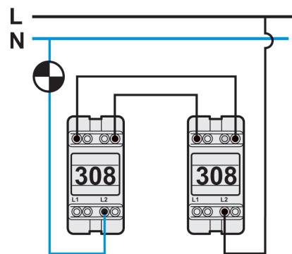
Va-et-vient
