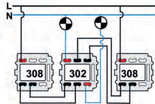
Double va-et-vient
