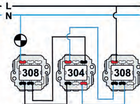
Permutateur
