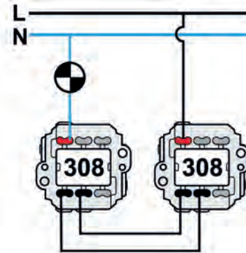
Va-et-vient
