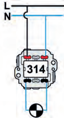
Interrupteur bipolaire
