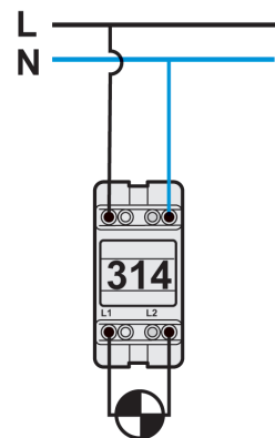
Interrupteur bipolaire
