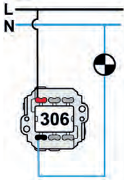
Interrupteur
