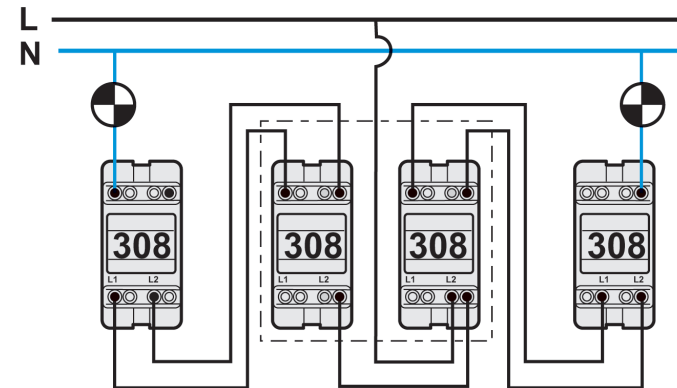
Double va-et-vient
