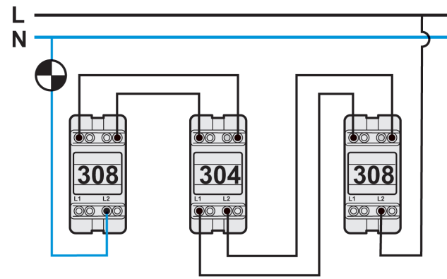
Permutateur
