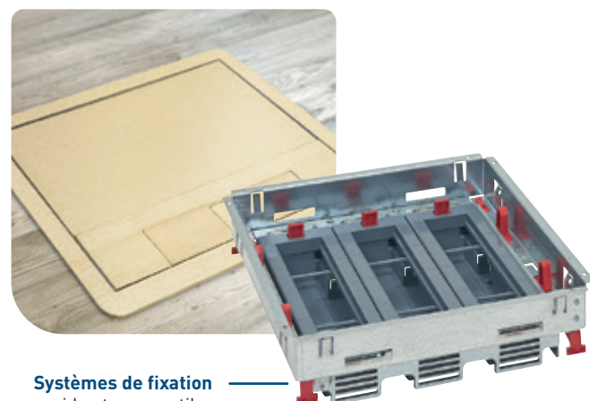
Pieds réglables pour ajuster parfaitement l'aplomb et la hauteur de la boîte
